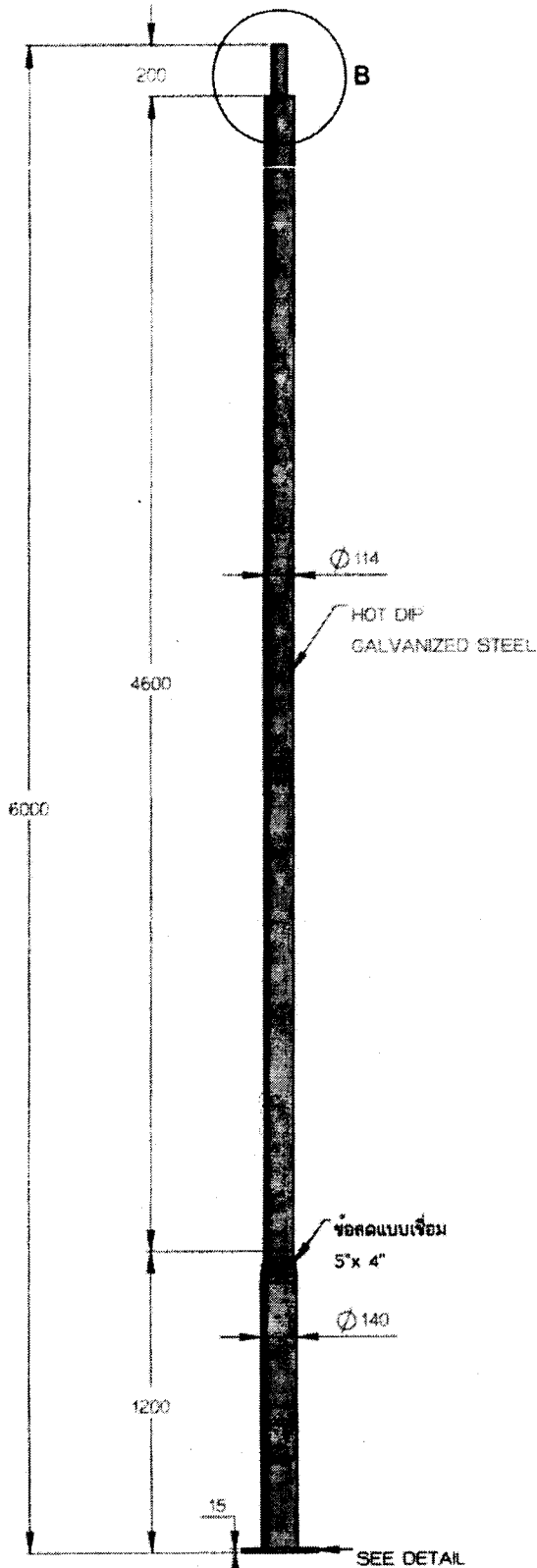
HI-WC5-060 เสากลมสูง 6 เมตร ขนาด 5 นิ้ว กว้าง 4 นิ้ว SCALE 1 : 28
